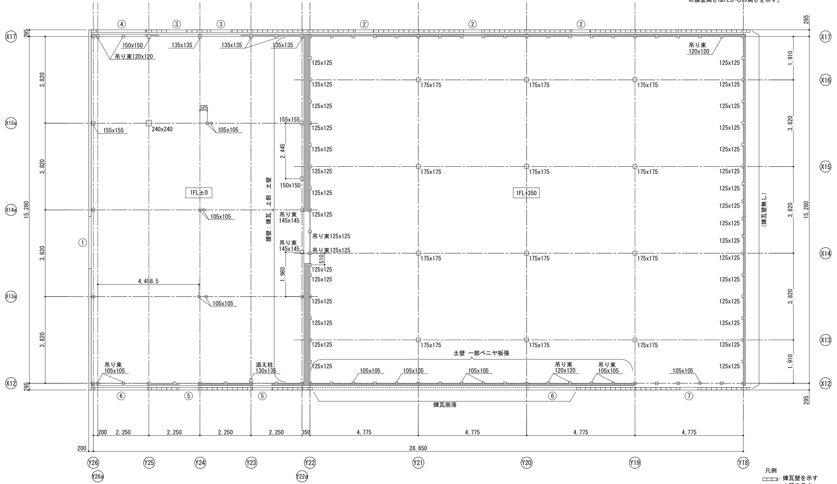
1階柱壁伏図
