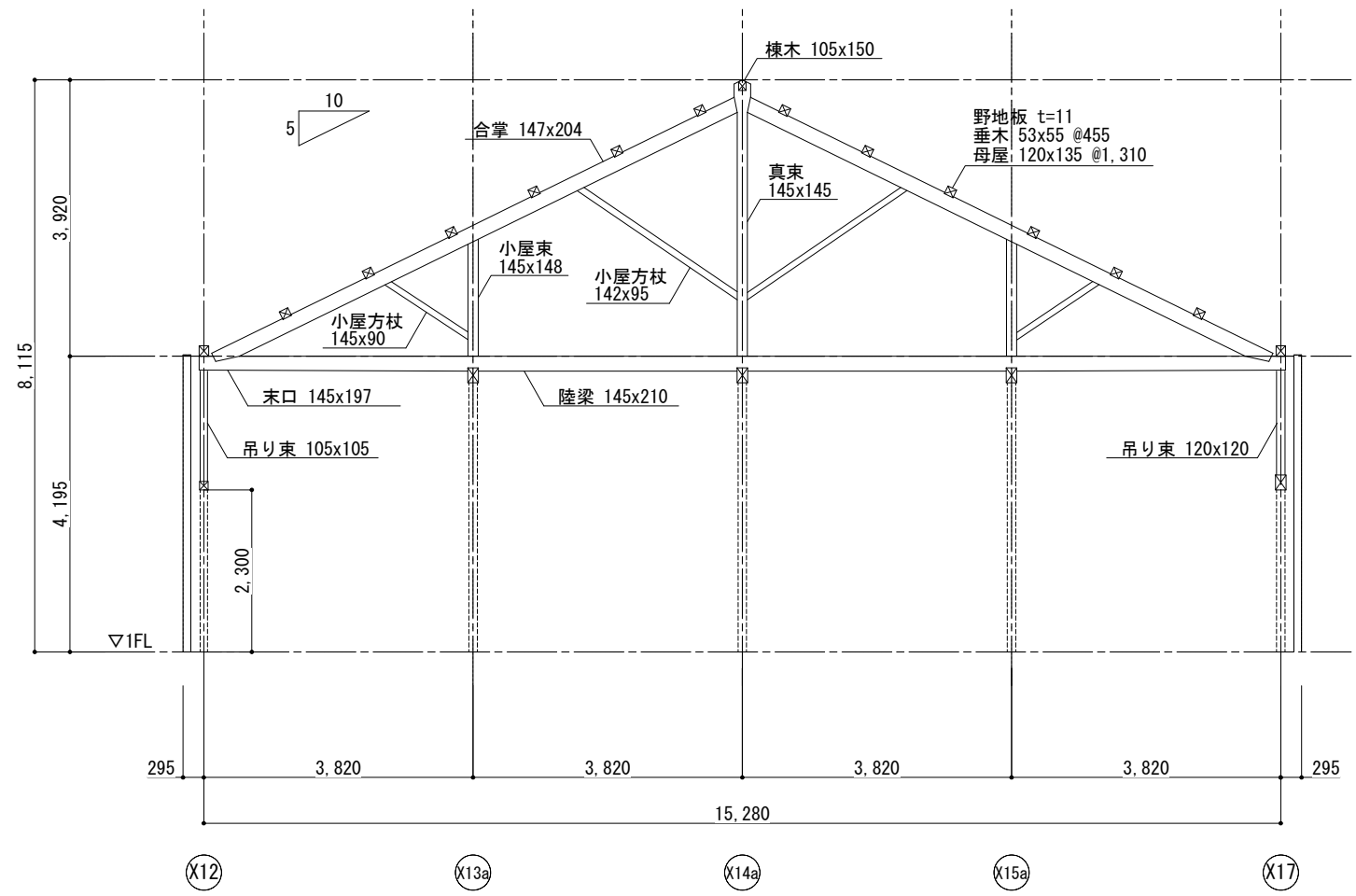
Y26a通り軸組図
