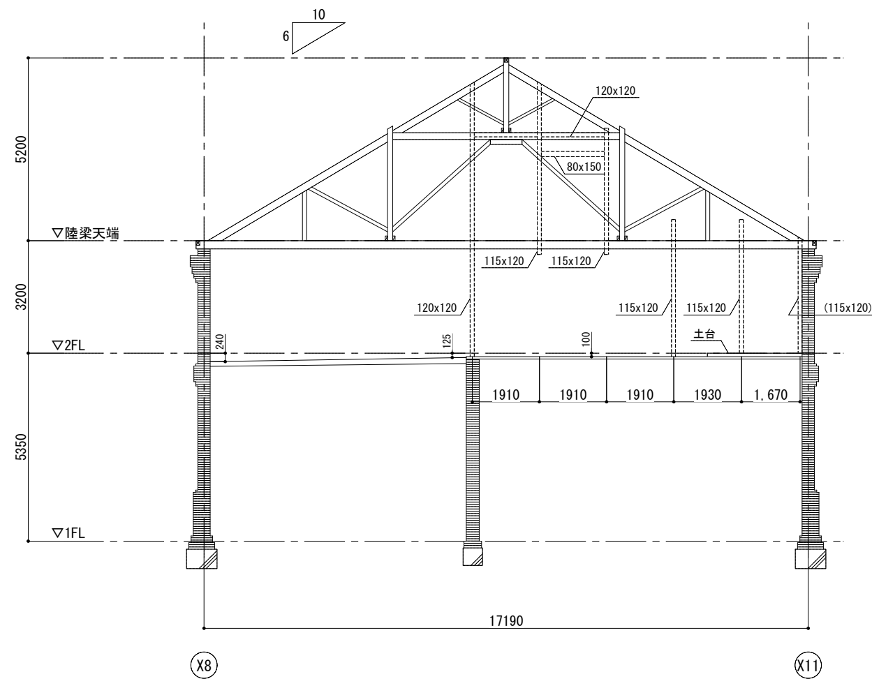
Y10通り軸組図
