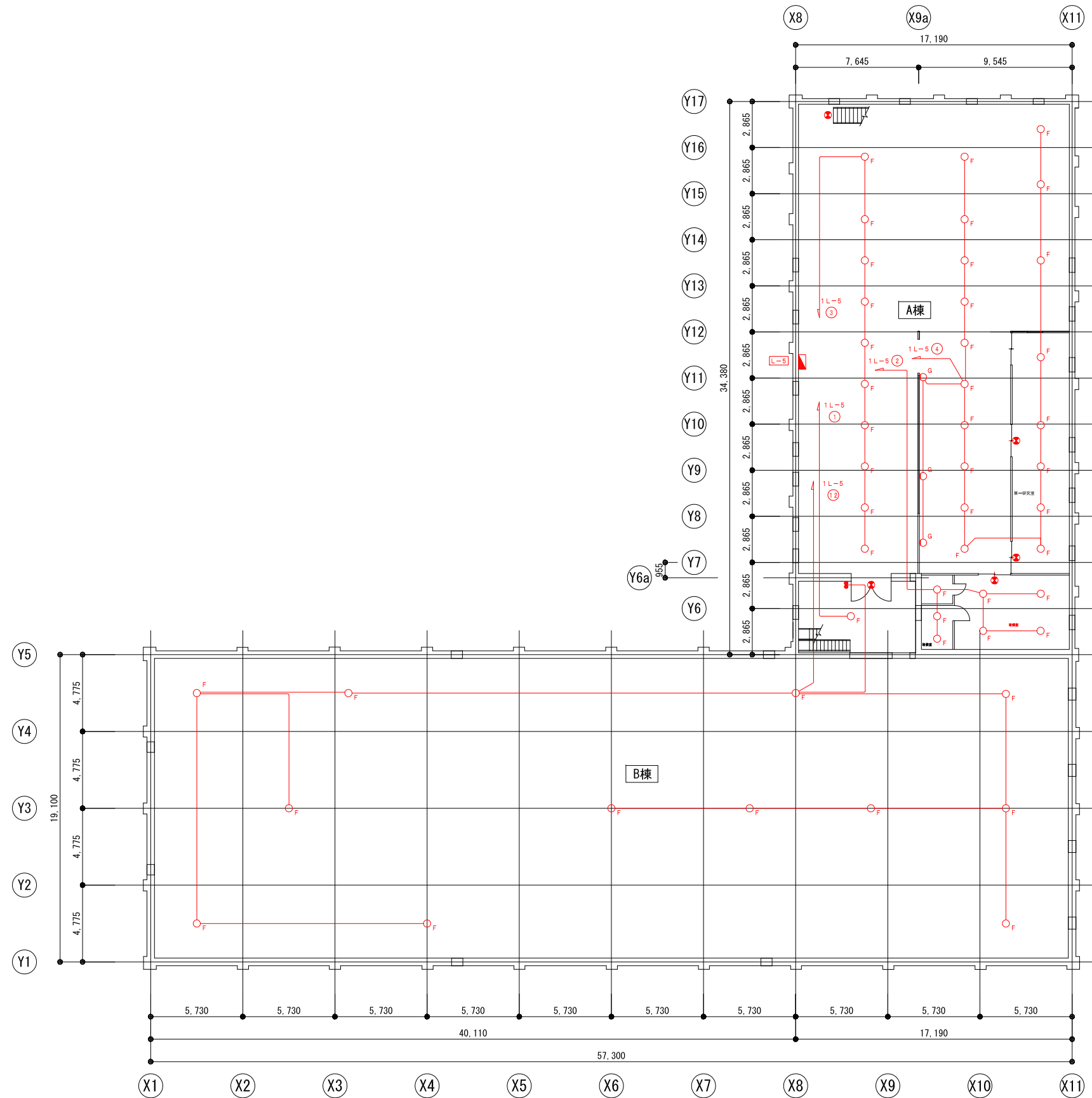
2階柱壁伏図
