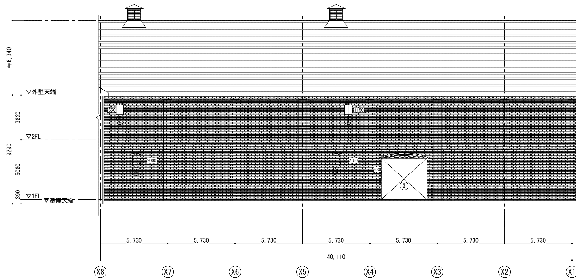
西側立面図
