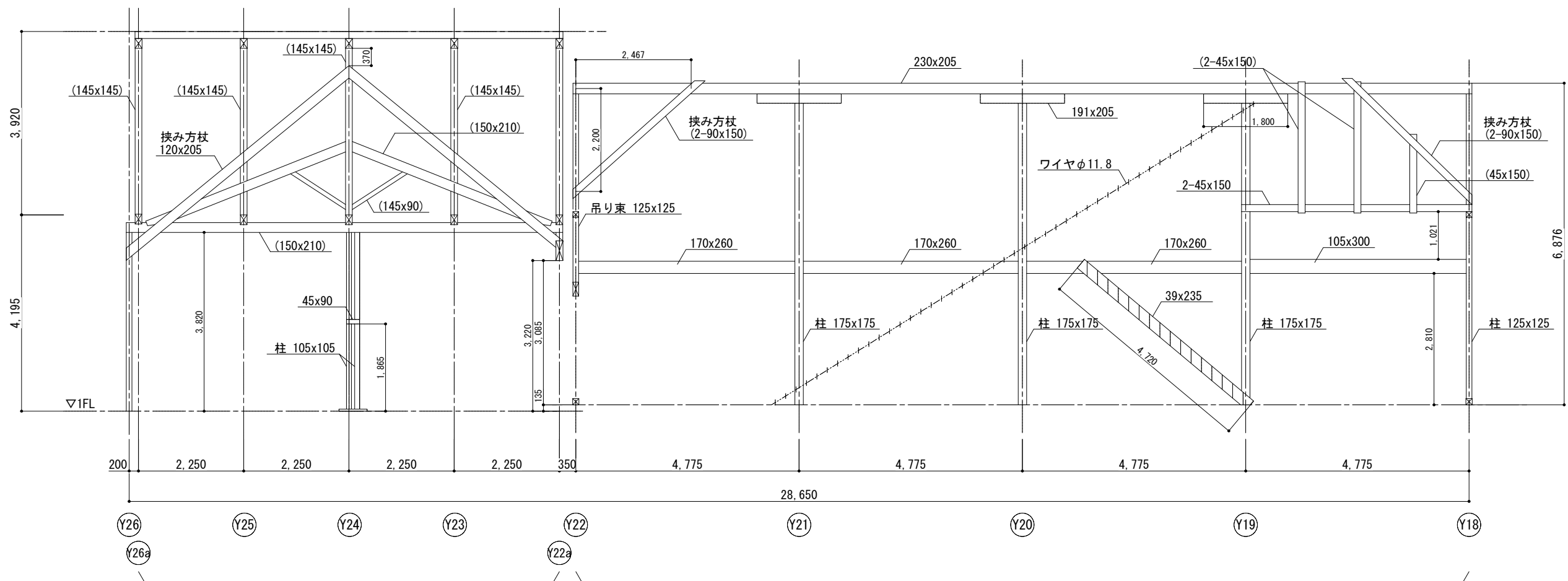
X14a通り軸組図
