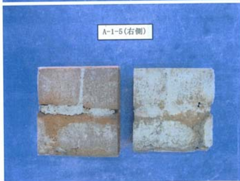
写真-62 目地モルタルの破壊状況 (写真-60 右側) [A-1-5]
