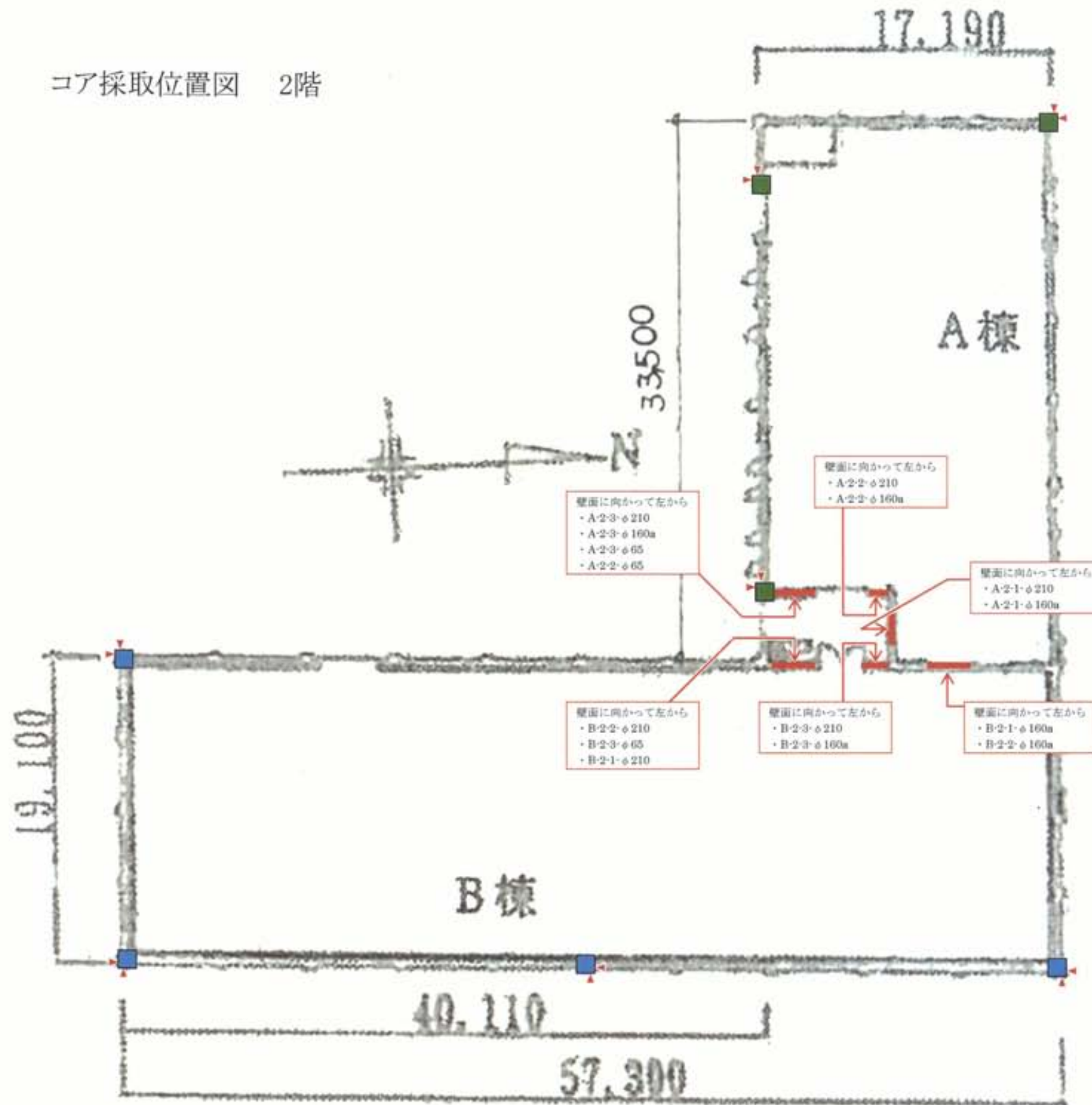
2階平面図
