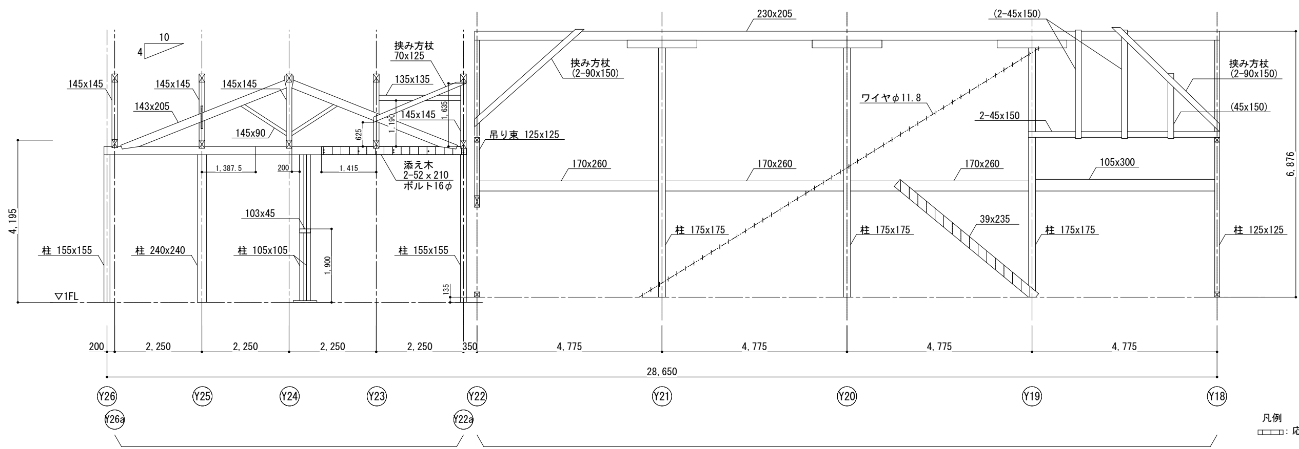
X15a通り軸組図
