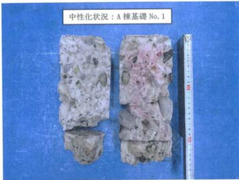
写真-4 中 性 化 状 況 [A棟基礎No. 1]
