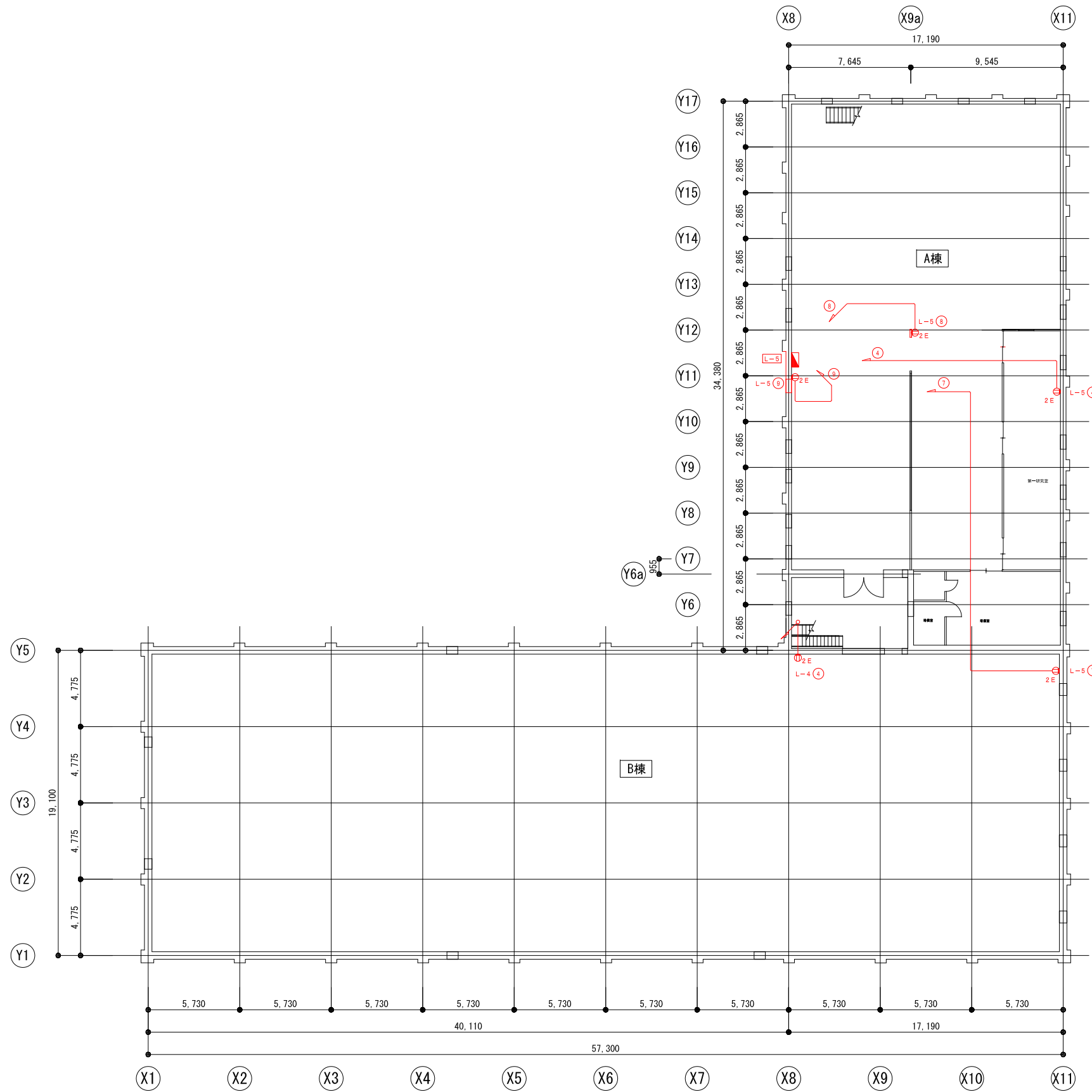
2階柱壁伏図
