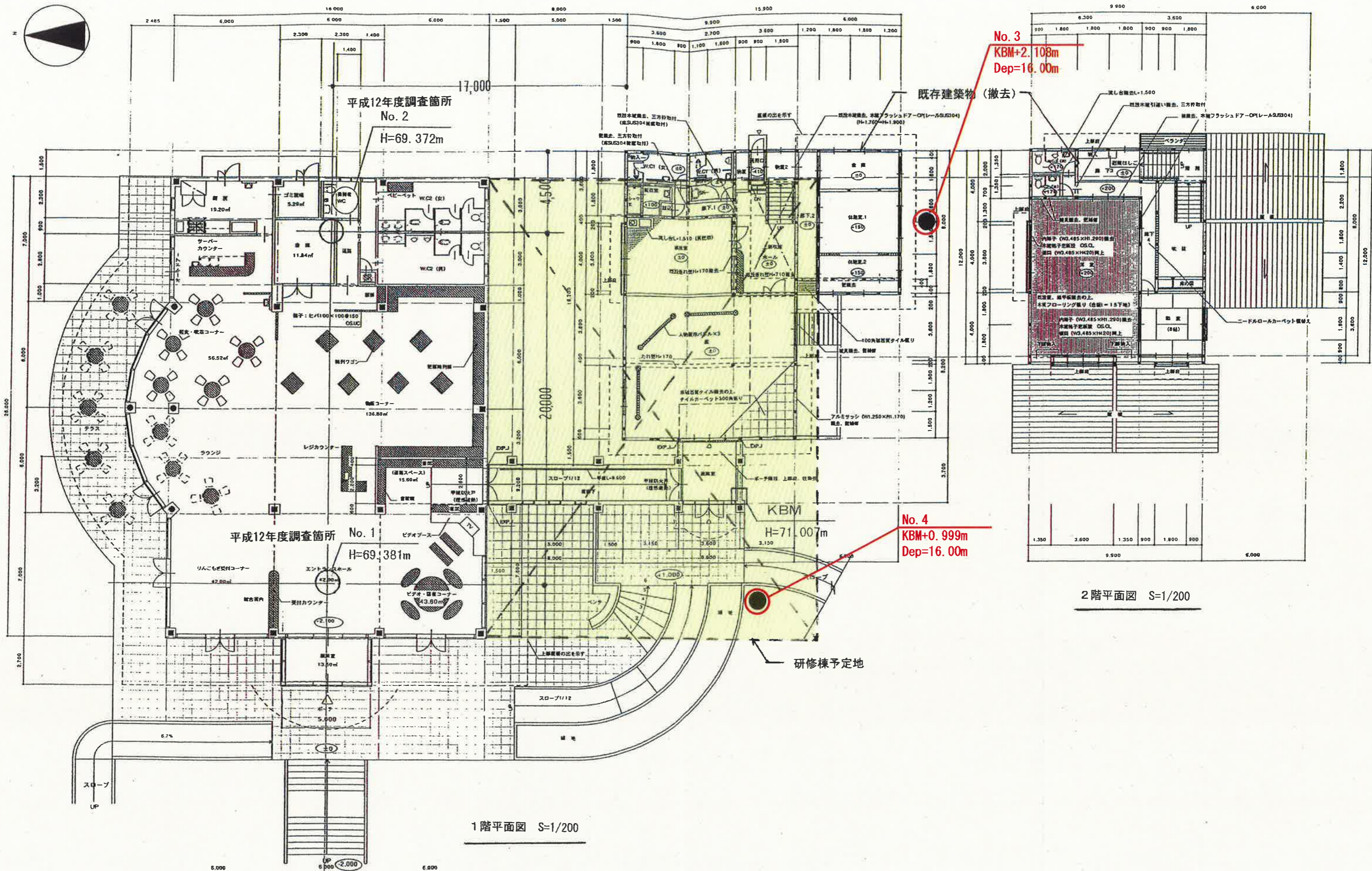
図 4-1(2) 調査位置平面図(研修棟) S=1:200
