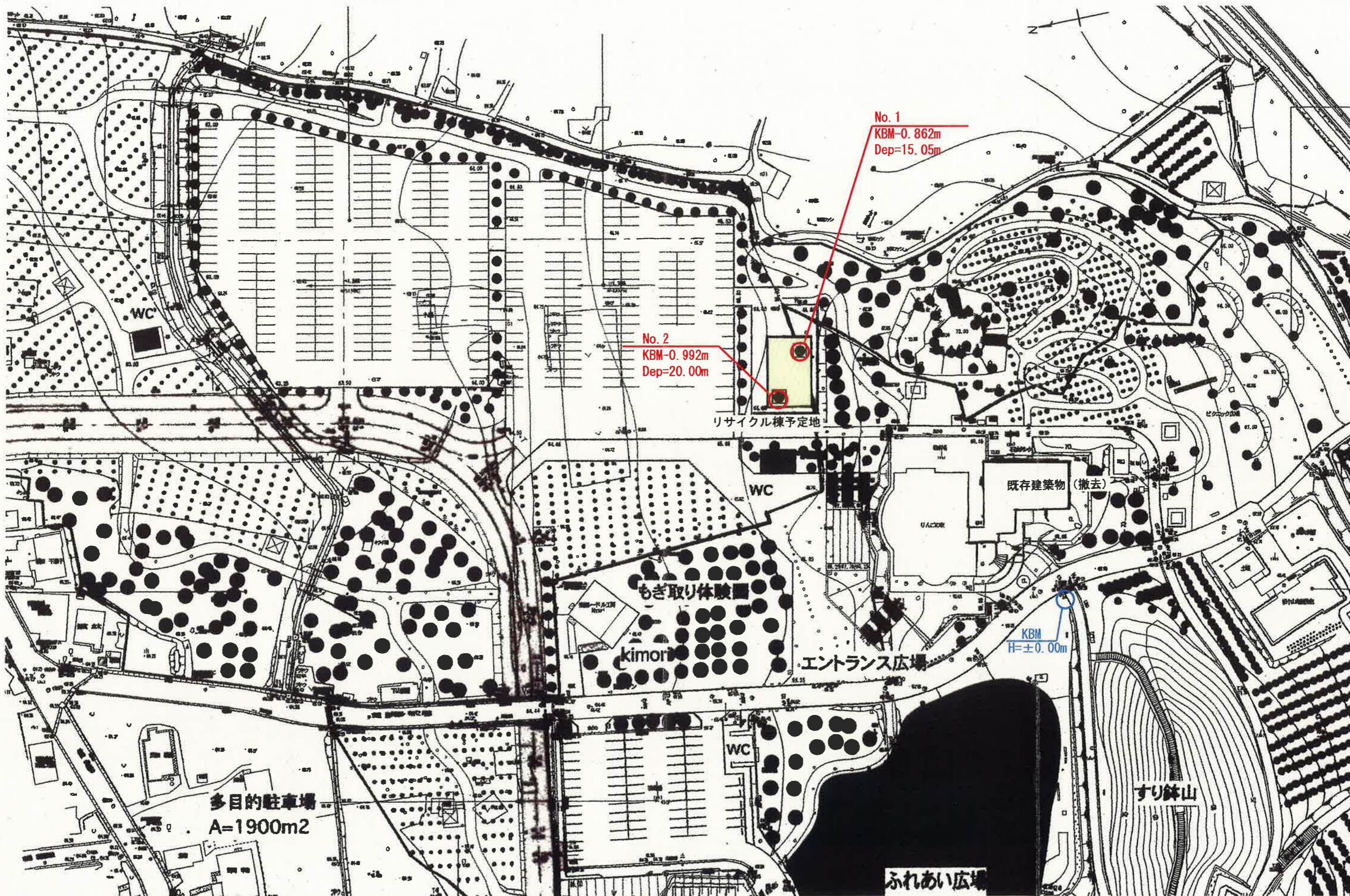
図 4-1(1) 調査位置平面図(リサイクル棟) S=1:1,000
