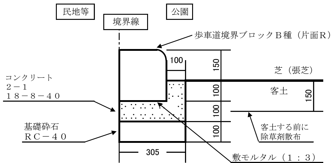
図4 公園、緑地用地の縁石及び緑化整備（第13条第1項第5号、第6号関係）
