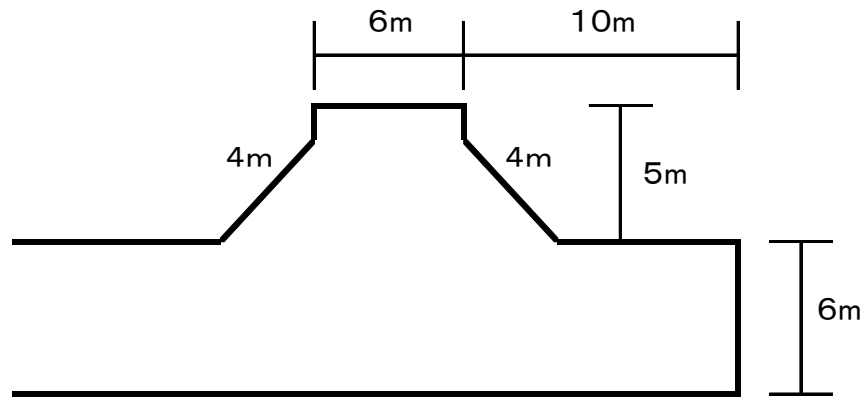
図3 袋路状道路に設ける転回広場（第12条第1項第5号関係）
