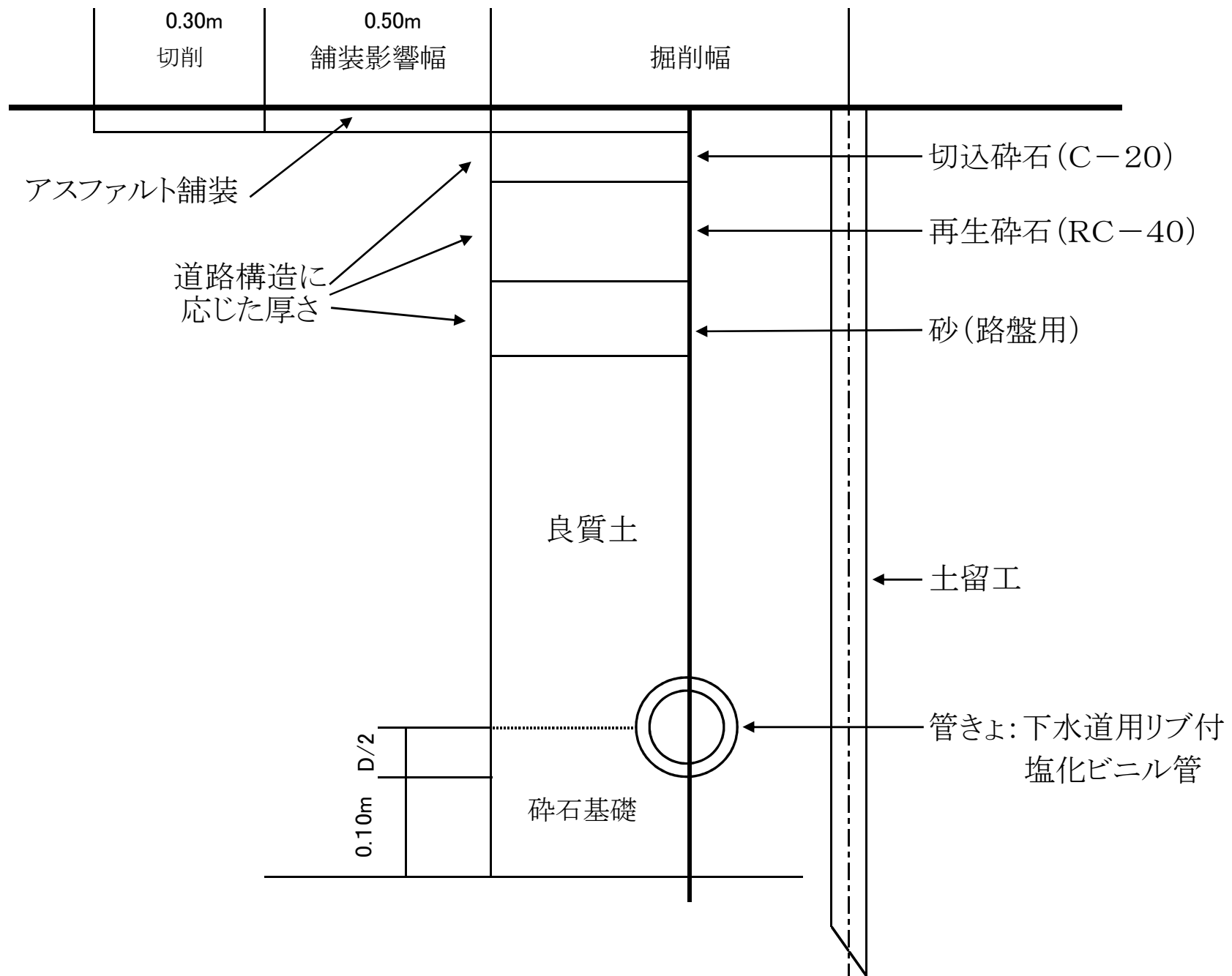
図5 管きよ布設の標準断面(第15条第3項第4号関係)
