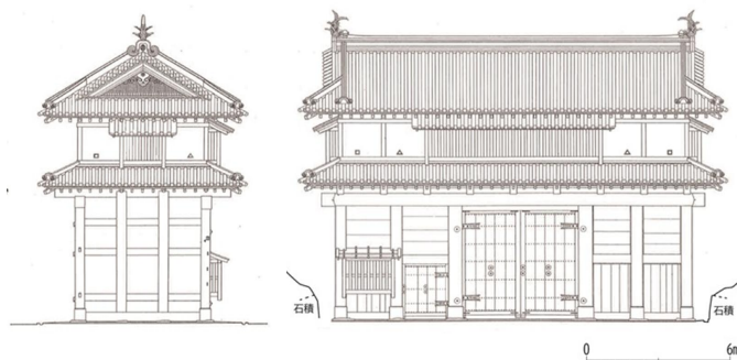
【図2】二の丸東門立立面図
