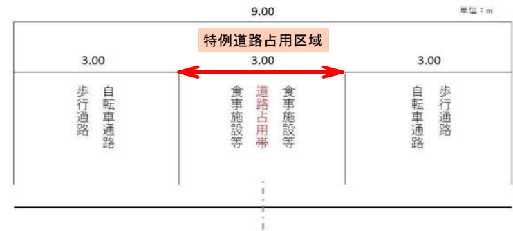
断面図
